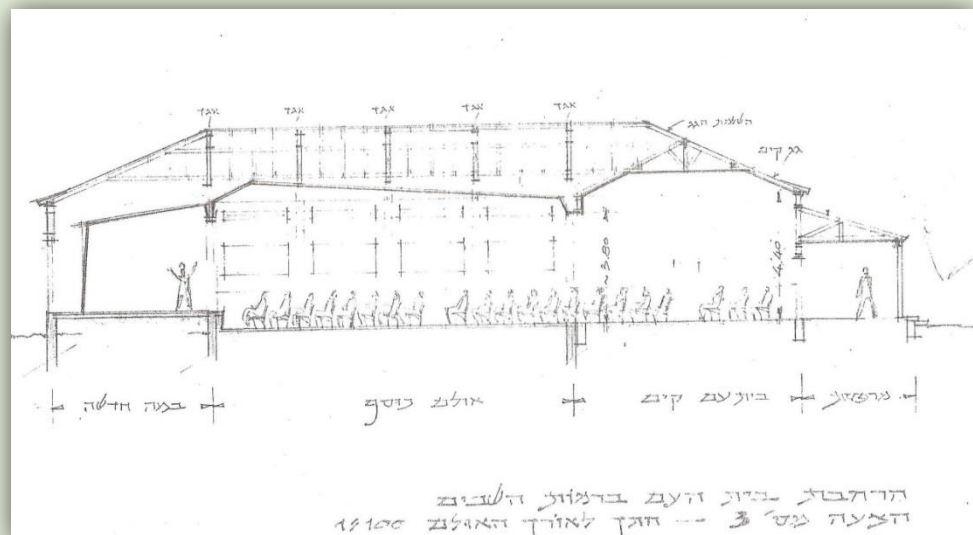
איור 1: חתך רוחב של האולם, מבט ממזרח
